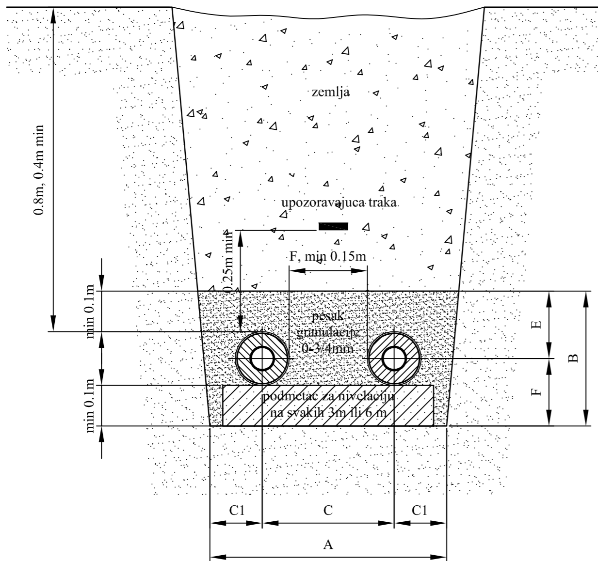
TOPLOVOD U ZELENOJ POVRŠINI
