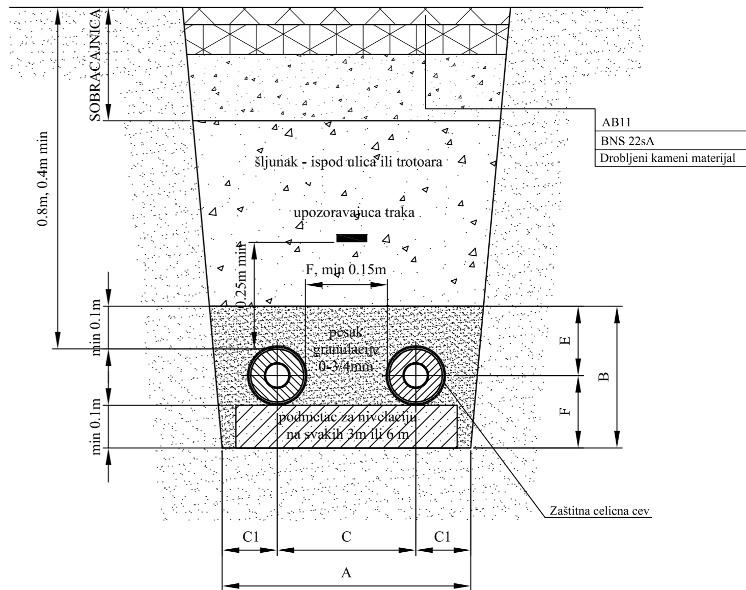
TOPLOVOD ISPOD SAOBRAČAJNICA
